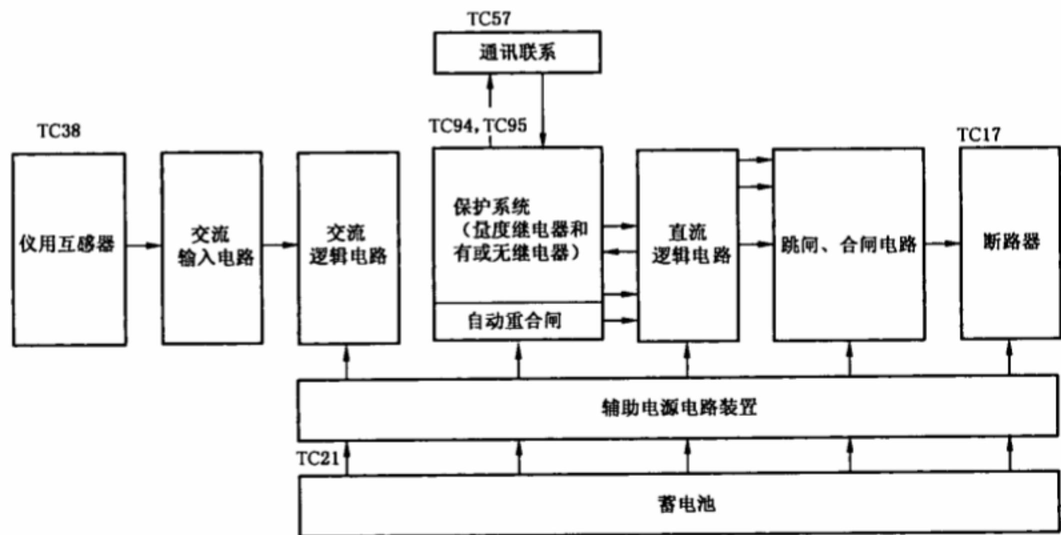
附录 A (资料性附录) 保护系统方框图
